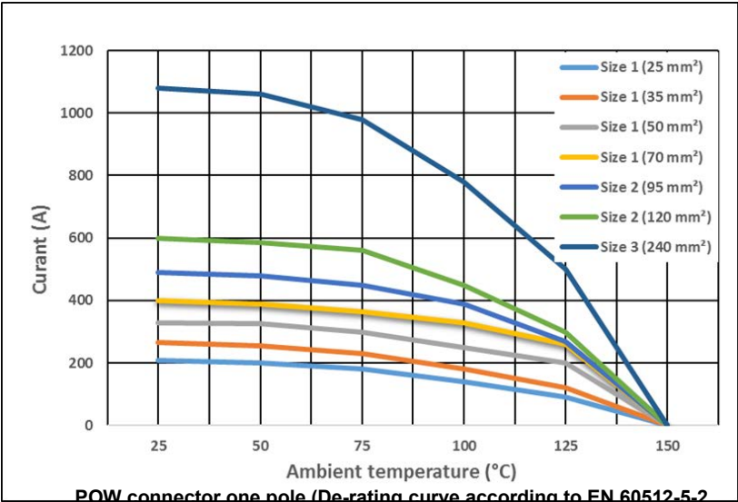
De-rating POW connector (EN 60512-5-2)
